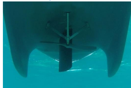
Quilles, hélice et safran
